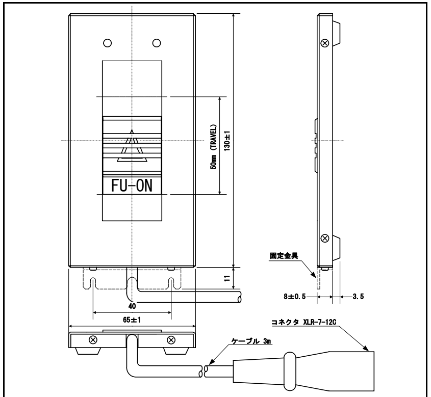
・外形図(図1)
